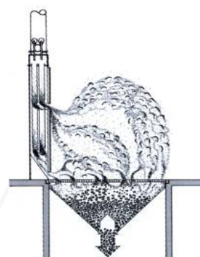
Двухщелевое приемное устройство
